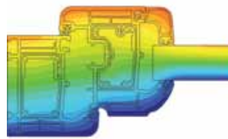
Termografía Zendow#neo standard marco 5001 (ref. 5202) + hoja 3146 (ref. 5220)
